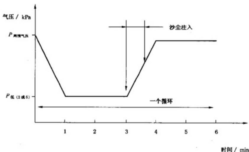
图 2 试验箱内的气压循环——类型 1
