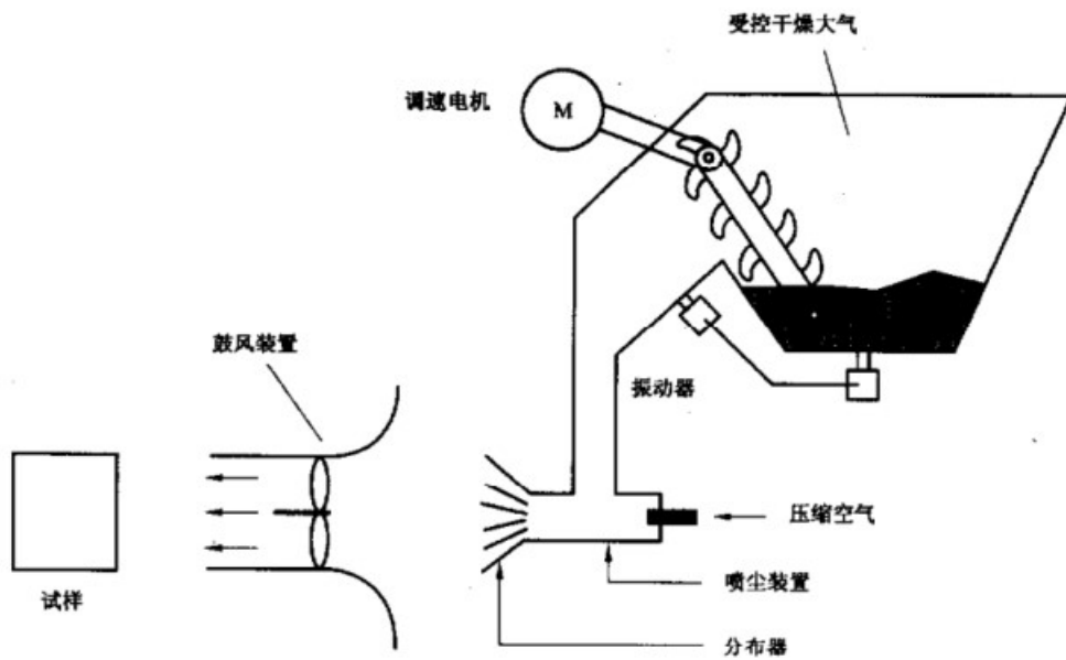
图7 方法 Lc2 适用的喷尘系统实例
