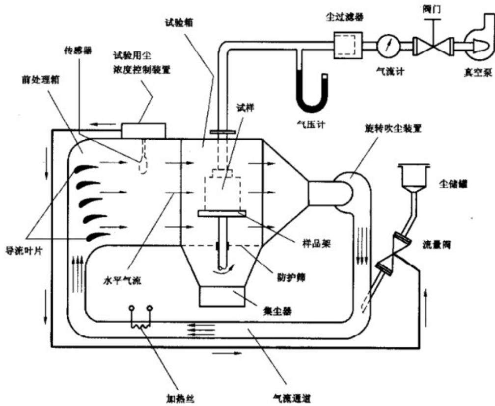
图6 方法 Lc1 适用设备的基本布置图
